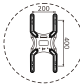
VESA 200x400
