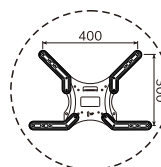
VESA 400x300
